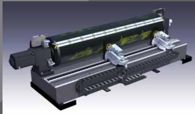
Diseño modular con doble cabezal en TFxX 60 y 80.
