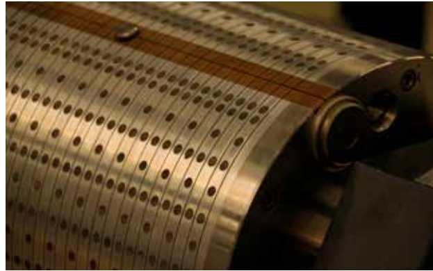
Tambor híbrido para planchas de flexografía y tipografía de tipo Steel back.
